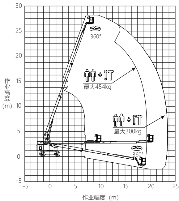
LT26JG4性能曲线图
